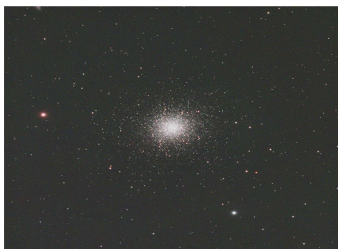
ヘルクレス座の球状星団(M13)
