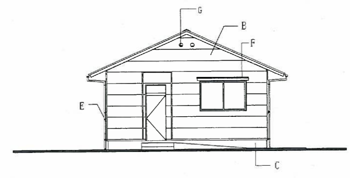
西立面図 1:100
