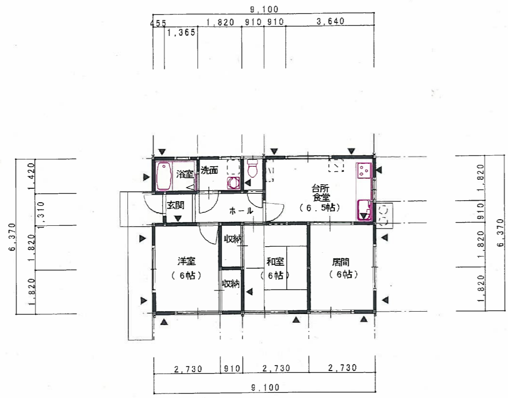
平面図
