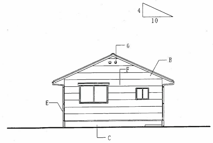
東立面図 1:100
