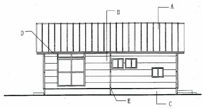
北立面図 1:100
